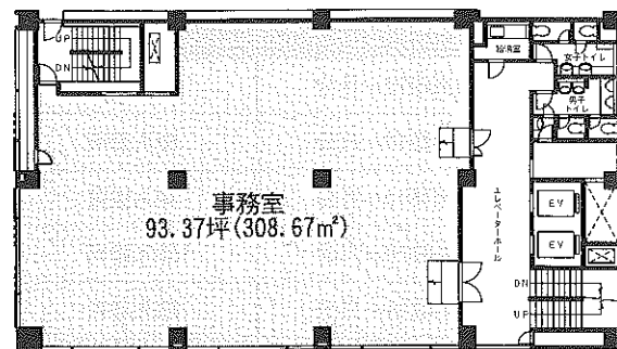
3階平面図
