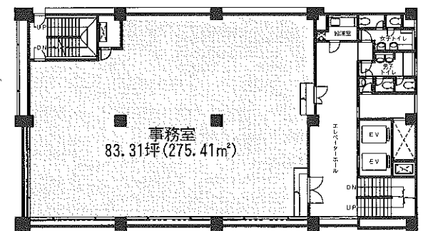
0階平面図
