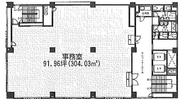
6階平面図
